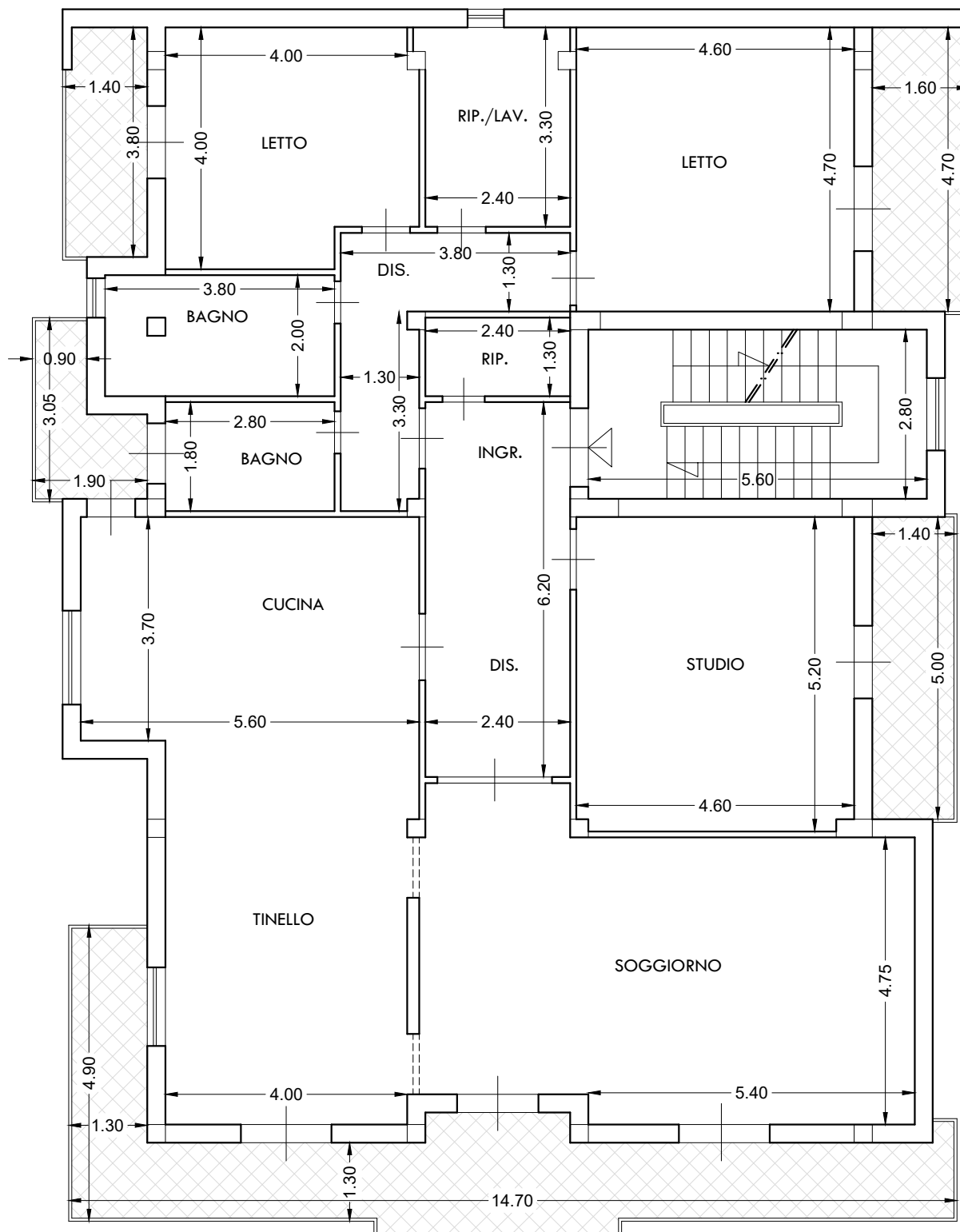
PIANO PRIMO - rapp. 1:100
