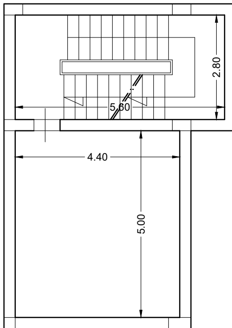
PIANO INTERRATO - rapp. 1:100
